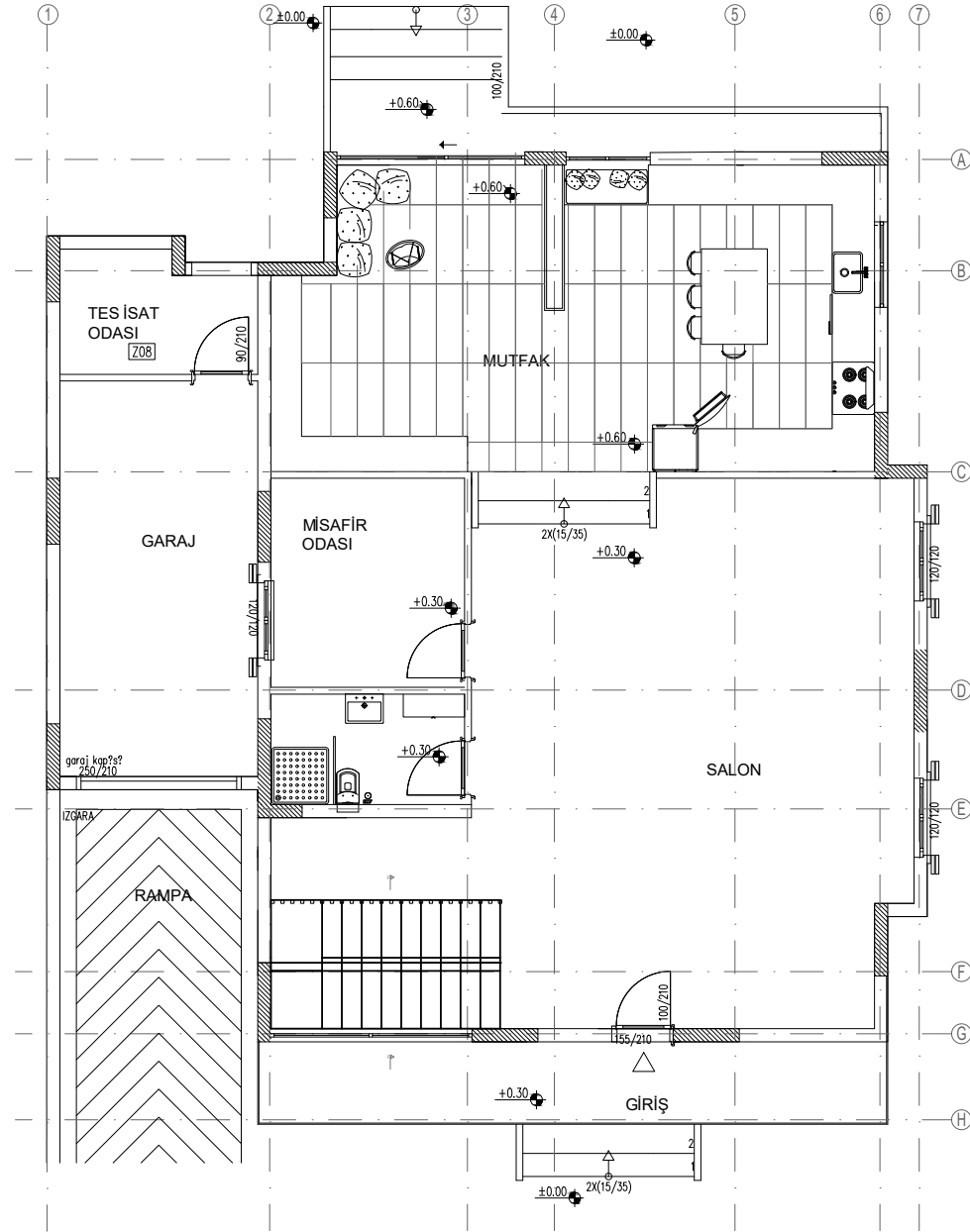
GİRİŞ KAT PLANI 1/50
