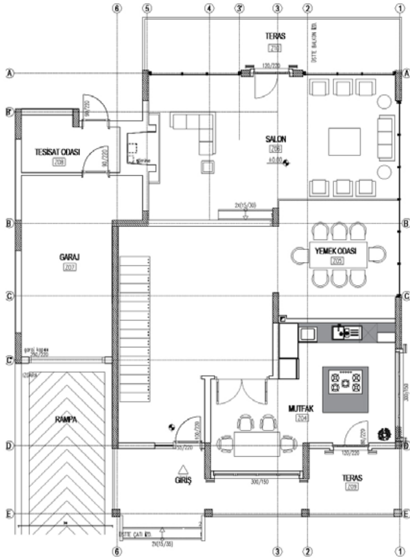
ZEMİN KAT PLANI
