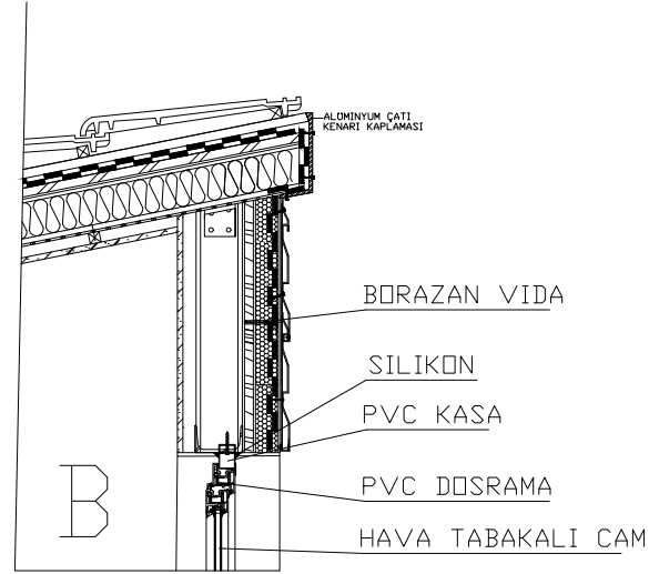
YALI BASKISI DİS CEPHE KAPLAMASI
